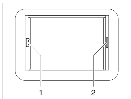
Afb. 53 Heki-dakluik, rolgordijn-vergrendeling
