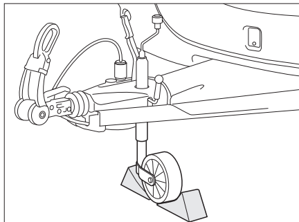
Afb. 161 Steunwiel beveiligen
