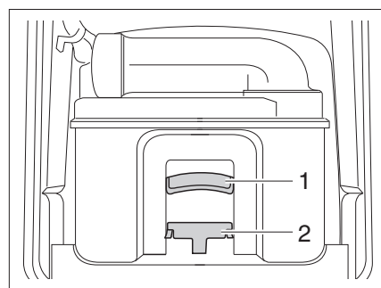
Afb. 146 Thetford-cassette
