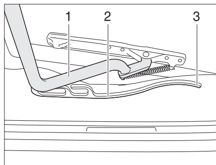
Afb. 47 Heki-dakluik, geleiding
