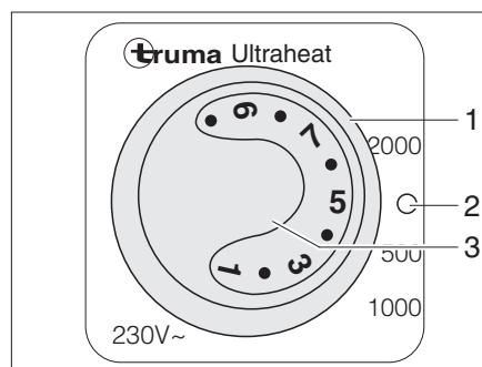
Afb. 116 Bedieningsgedeelte elektrische extra verwarming Ultraheat
