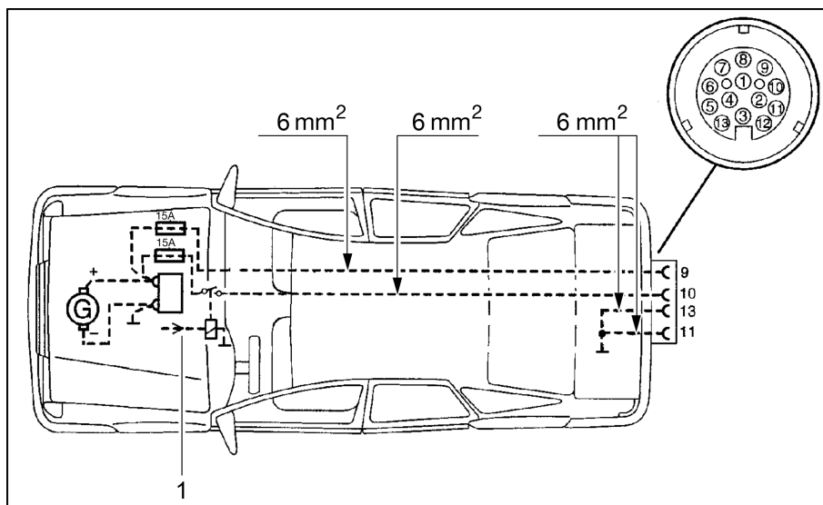
Afb. 102 Trekwagen-installatieschema
