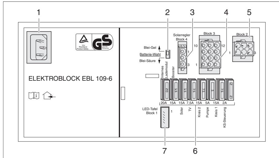
Afb. 93 Elektroblok EBL 109
