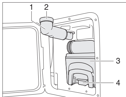
Afb. 143 Thetford-cassette
